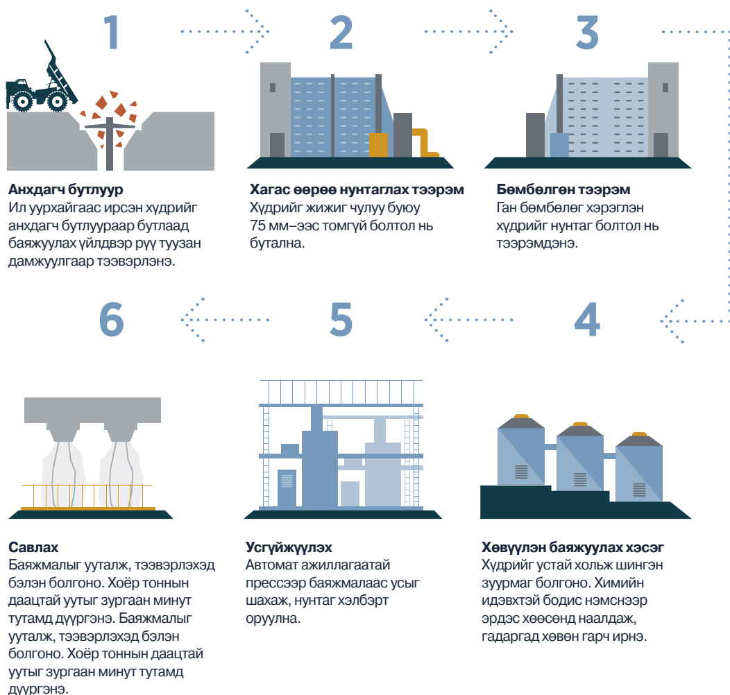
Зураг 8. Баяжуулах үе шат
