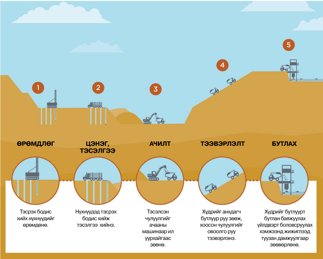
Зураг 7. Ил уурхайн олборлолтын үйл ажиллагаа
