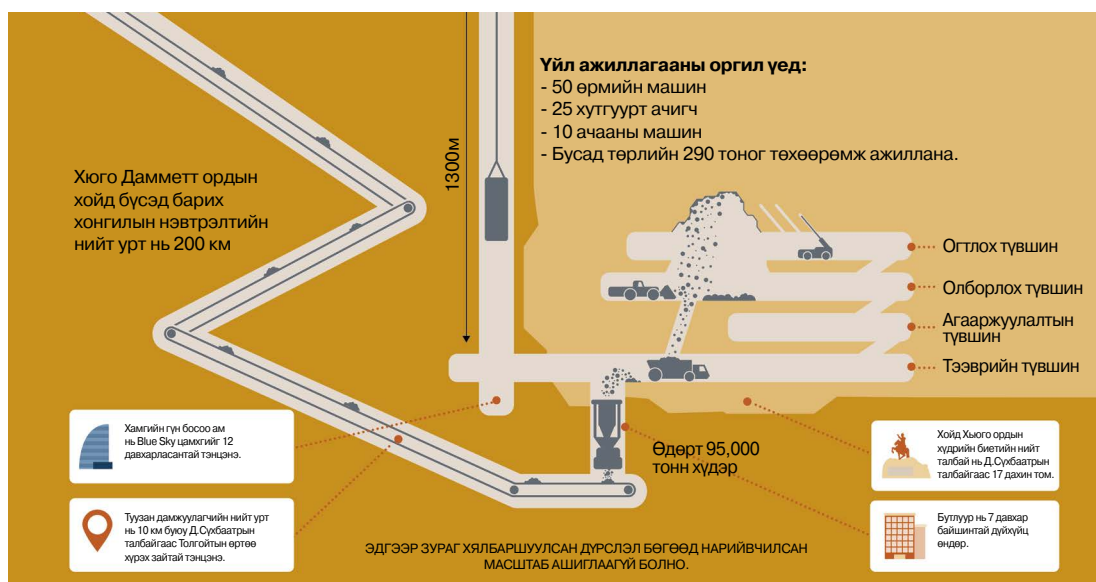
Зураг 9. “Оюу толгой”-н гүний уурхайн өргөтгөл
